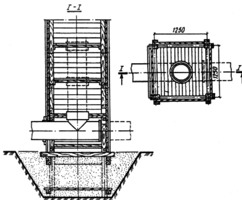
Рис. 6. Односекционный деревянный водосборной колодец с трубчатым стояком высотой св. 6 м
