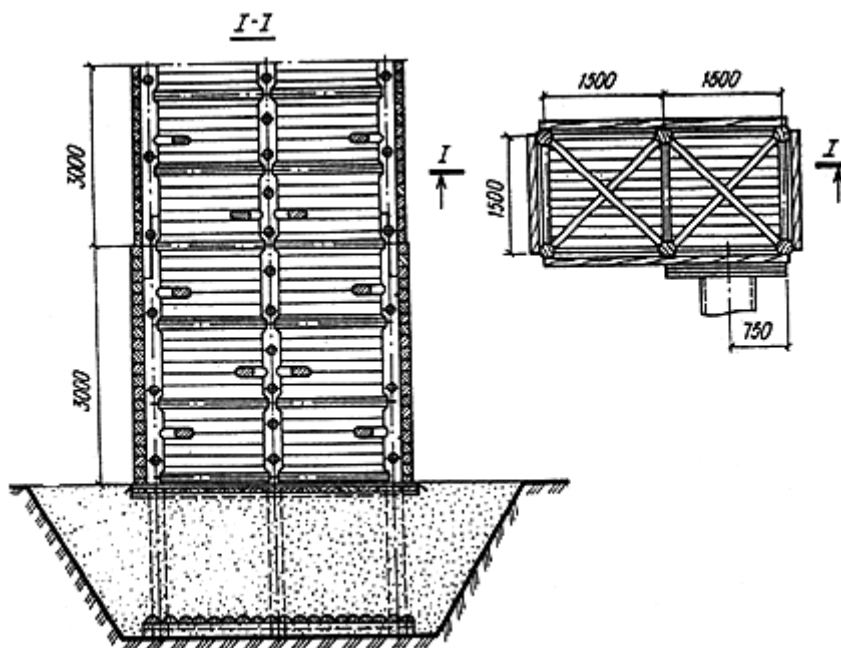
Рис. 9. Двухсекционный деревянный водосборной колодец высотой до 6 м
