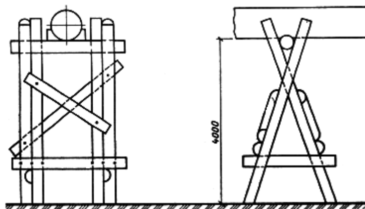
Рис. 5. Козловая опора
