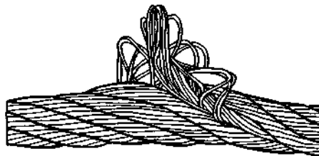
Рис. 4. Выдавливание сердечника
